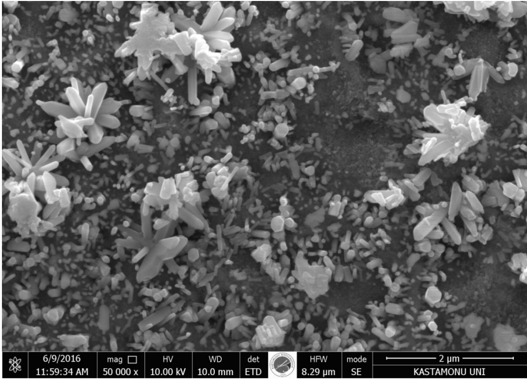
Şekil 5.8. Zn_{97}Er_{3}O ince filmlerine ait farklı kaplama kalınlıklarındaki a) 10 dip, b) 15 dip ve c) 20 dip SEM görüntüleri.
