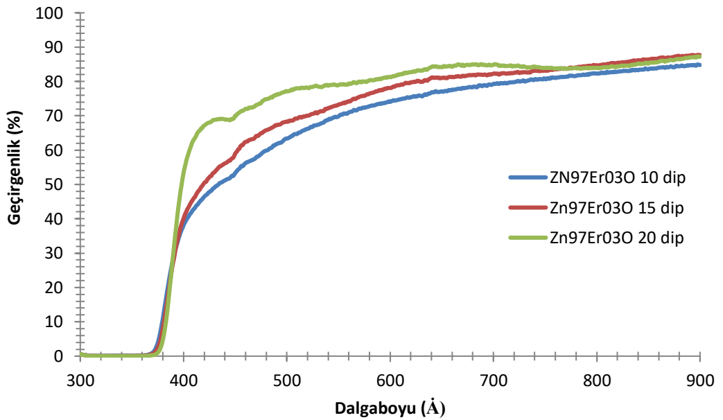
Şekil 5.20. Zn97Er03O ince filmine ait Geçirgenlik-Dalgaboyu değişimi
