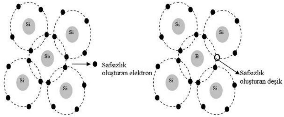
Şekil 2.2. a) n-tipi ve b) p-tipi yarıiletkenlerde bağ oluşumu
