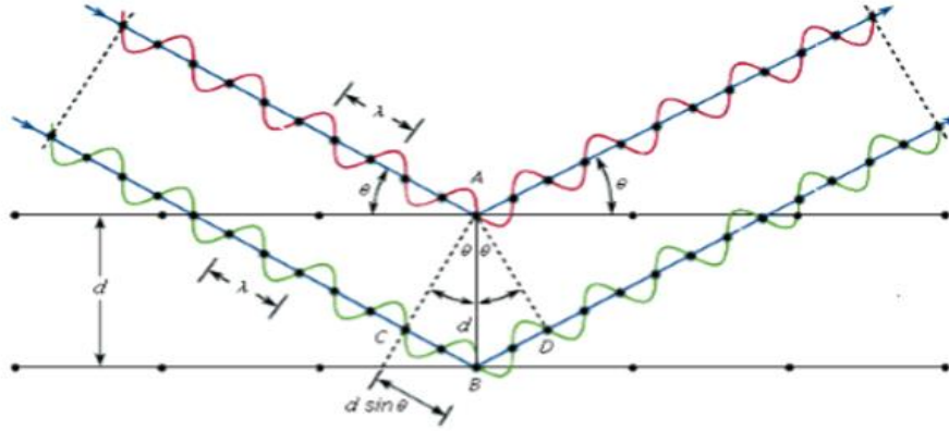
Şekil 2.5. Bragg yasası
