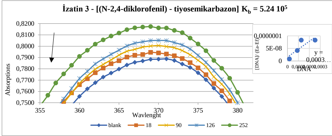
Şekil 4. 31. CT-DNA yokken İzatin 3 - [(N-2,4-diklorofenil) - tiyosemikarbazon]'un spektral absorbansı (--) ve (—) CT-DNA varlığında CT-DNA miktarında artış durumundaki değeri. Bileşik = 40 \mu M. Siyah ok ( \downarrow ) artan CT-DNA konsantrasyonları ile absorbanstaki değişimi gösterir.
