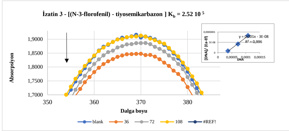
Şekil 4. 27. CT-DNA yokken İzatin 3 - [(N-3-florofenil) - tiyosemikarbazon 'un spektral absorpsiyonu (--) ve ( )CT-DNA varlığında CT-DNA miktarında artış durumundaki değeri. Bileşik = 40 \mu M. Siyah ok (↓) artan CT-DNA konsantrasyonları ile absorbanstaki değişimi gösterir.
