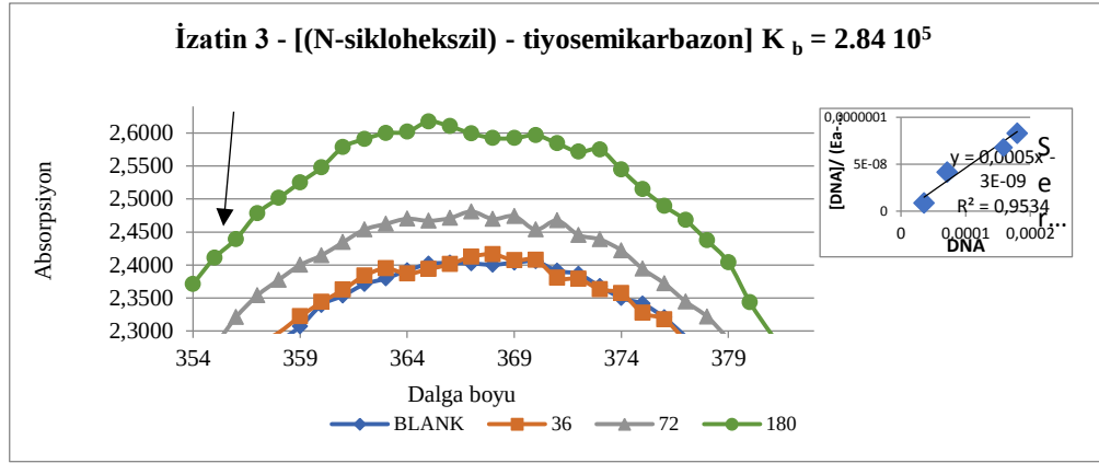
Şekil 4. 32. CT-DNA yokken İzatin 3 - [(N-siklohekszil) - tiyosemikarbazon]'un spektral absorbansı (--) ve (—)CT-DNA varlığında CT-DNA miktarında artış durumundaki değeri. Bileşik = 40 \mu M. Siyah ok ( \downarrow )artan CT-DNA konsantrasyonları ile absorbanstaki değişimi gösterir.
