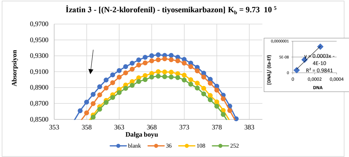
Şekil 4. 30. CT-DNA yokken İzatin 3 - [(N-2-klorofenil) - tiyosemikarbazon]'un spektral absorbansı (--) ve (—) CT-DNA varlığında CT-DNA miktarında artış durumundaki değeri. Bileşik= 40 \mu M Siyah ok (↓) artan CT-DNA konsantrasyonları ile absorbanstaki değişimi gösterir.
