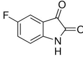
Şekil 1. 2. 5 - Floro-İzatinin Kimyasal Yapısı
