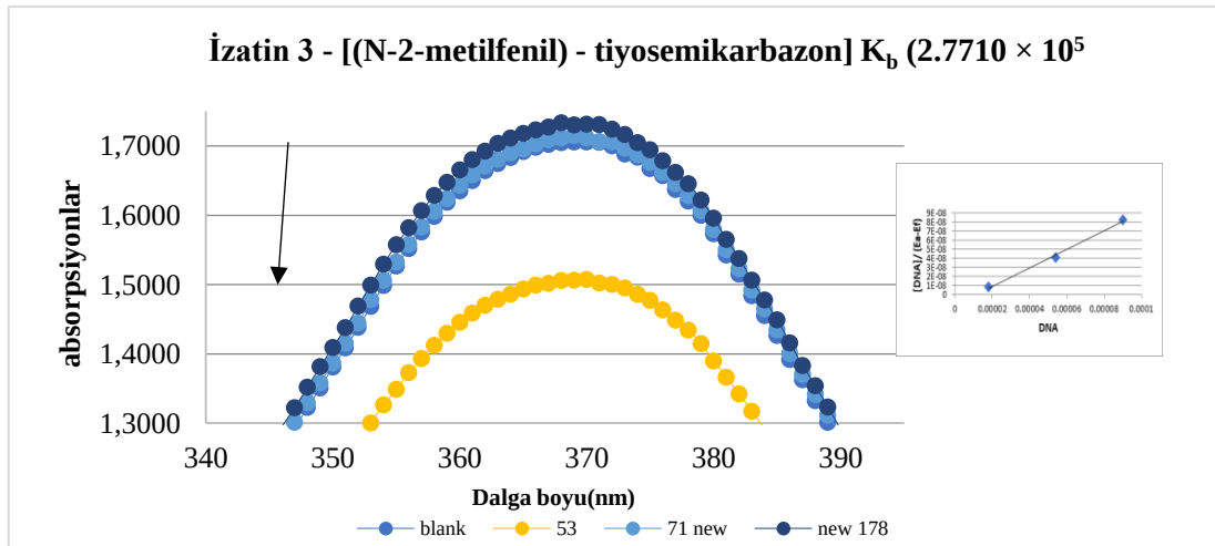
Şekil 4. 25. CT-DNA yokken İzatin 3 - [(N-2-metilfenil) - tiyosemikarbazon] 'un spektral absorbansı (--) ve (__)CT-DNA varlığında CT-DNA miktarında artış durumundaki değeri. Bileşik = 40 \mu M. Siyah ok (↓) artan CT-DNA konsantrasyonları ile absorbanstaki değişimi gösterir.
