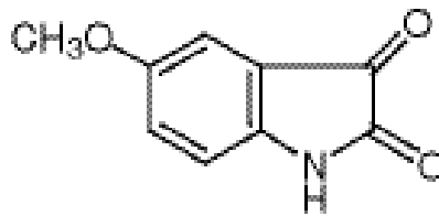
Şekil 1. 3. 5-Metoksi-İzatinin Yapısı
