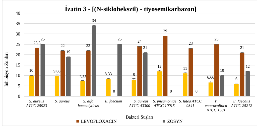
Şekil 4. 8. İzatin 3 - [(N-siklohekszil) - tiyosemikarbazon] 'un antimikrobiyal etkinliğı
