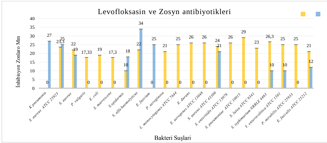
Şekil 4. 1. Levofloksasin ve Zosyn'in kullanılan bakterilere karşı antimikrobiyal etkinlikleri.
