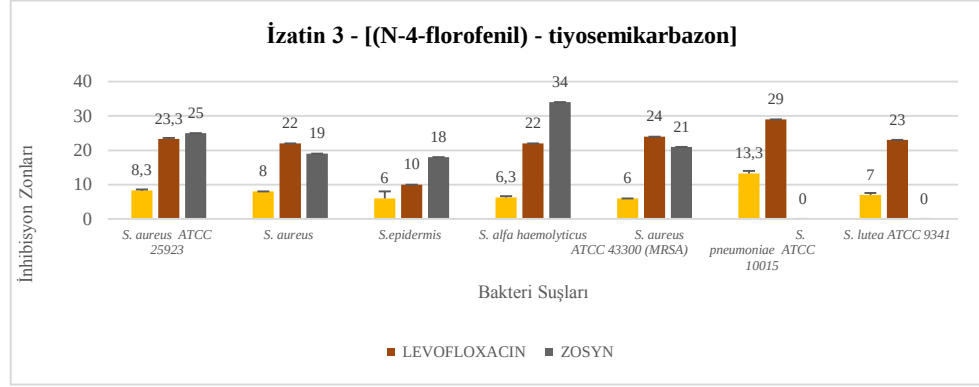
Şekil 4. 5. İzatin 3 - [(N-4-florofenil) - tiyosemikarbazon] 'un antimikrobiyal etkinliği
