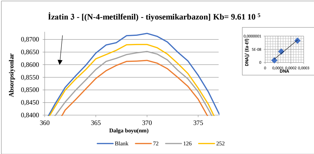
Şekil 4. 26. CT-DNA yokken İzatin 3 - [(N-4-metilfenil) - tiyosemikarbazon]'un spektral absorbansı (--) ve (—) CT-DNA varlığında CT-DNA miktarında artış durumundaki değeri. Bileşik = 40 \mu M. Siyah ok (↓) artan CT-DNA konsantrasyonları ile absorbanstaki değişimi gösterir.
