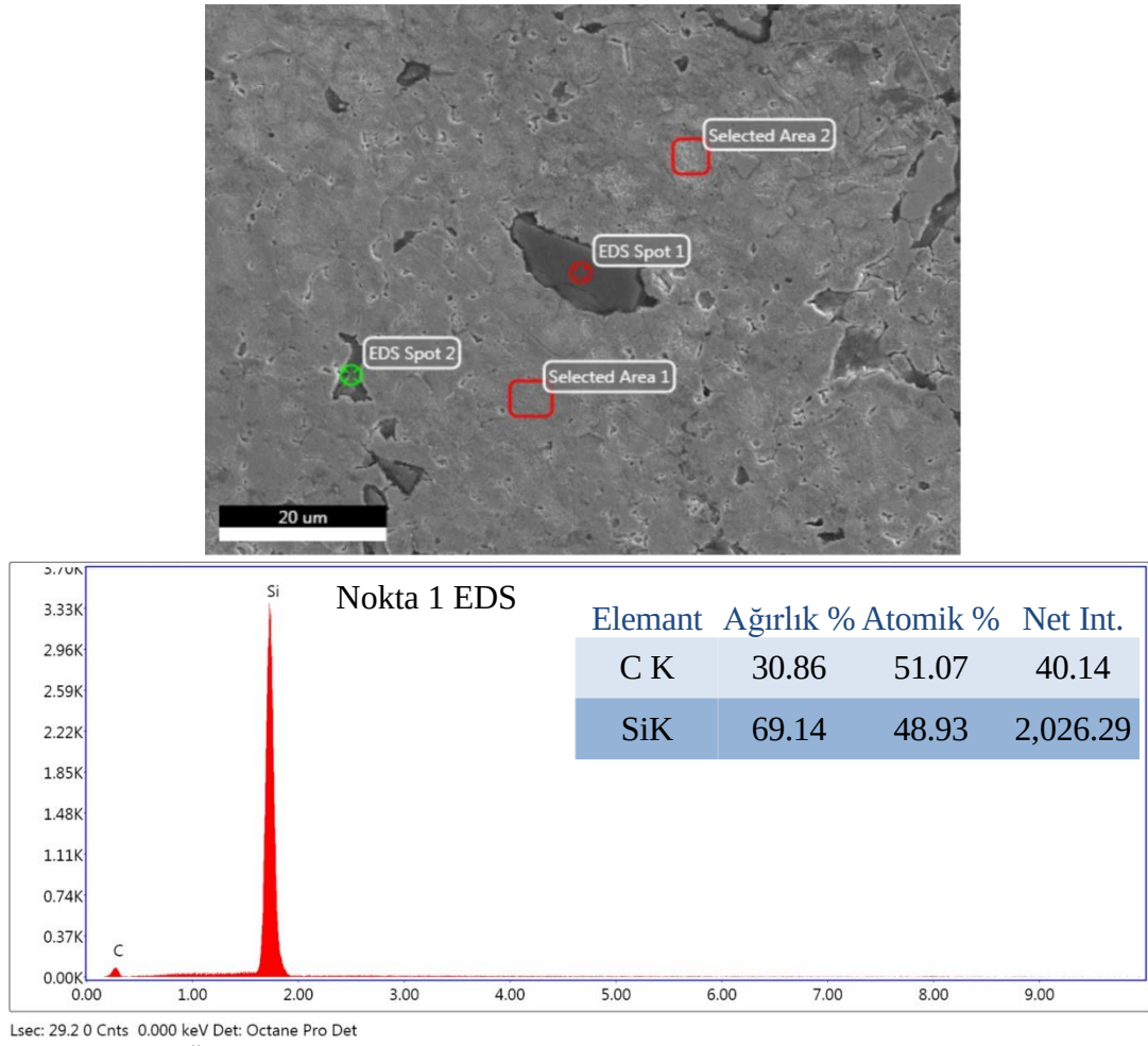
Şekil 6.8 Üretilen %1 SiC takviyeli CuNiSi kompozitinin SEM-EDS analiz sonucu
