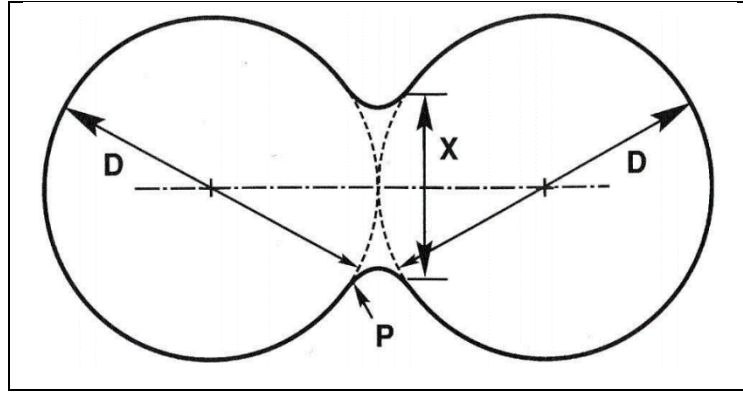
Şekil 4.10 İki tanenin sinterleme profili (Saritaş vd., 2007)
