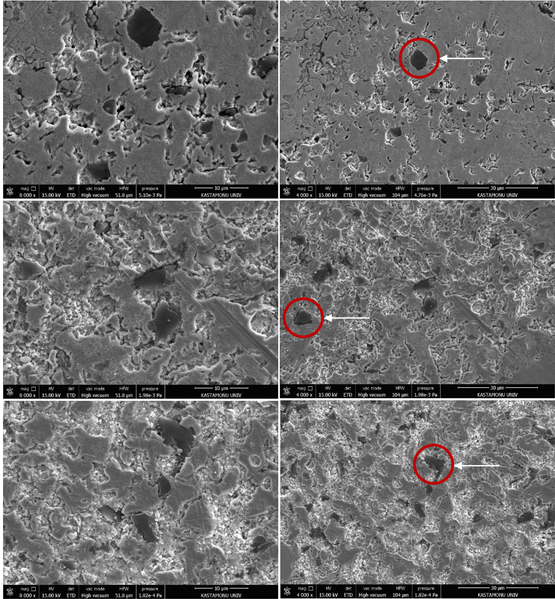
Şekil 6.2 Üretilen 2, 3 ve 4 numaralı numunelerin SEM görüntüleri
