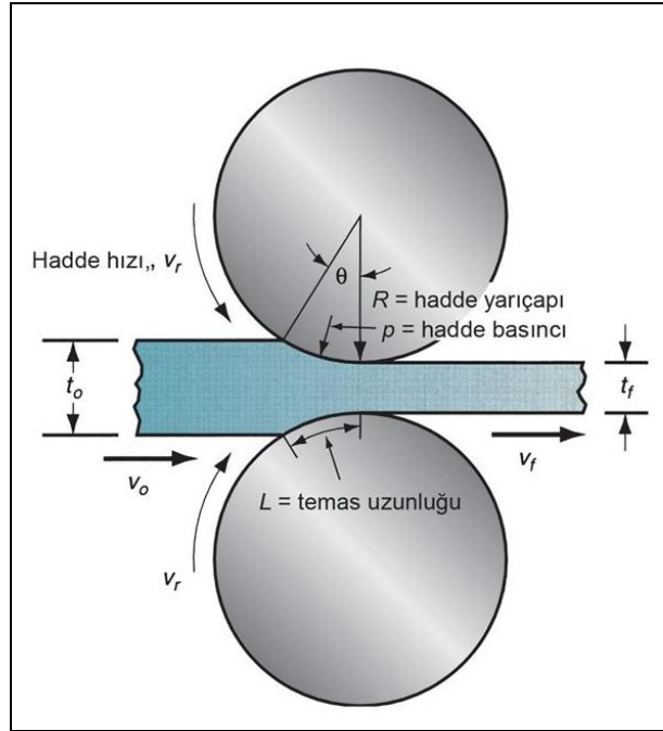
Şekil 4.4 Haddeme sistemi
