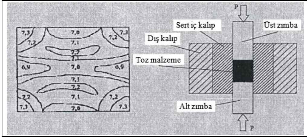
Şekil 4.6 Çift yönlü preslemede yoğunluk dağılımı ve çift yönlü kalıbın şematik gösterimi (Bahçeci, 2006; Matik, 2010)
