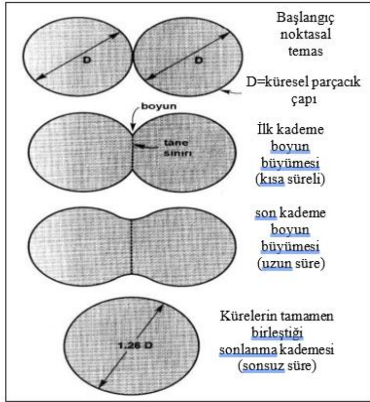
Şekil 4.11 İki tanenin sinterleme modeli
