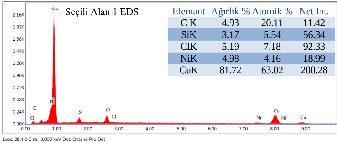
Şekil 6.10 Üretilen %5 SiC takviyeli CuNiSi kompozitinin SEM-EDS analiz sonucu
