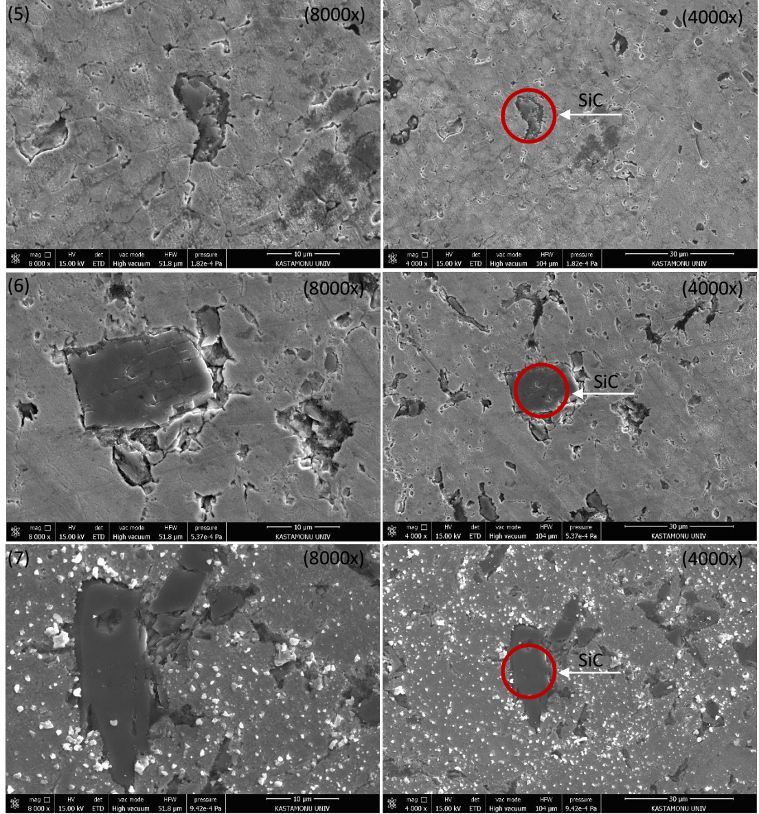
Şekil 6.3 Üretilen 5, 6 ve 7 numaralı numunelerin SEM görüntüleri
