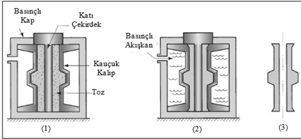
Şekil 4.7 Soğuk izostatik presleme şematik gösterimi (Bahçeci, 2006)
