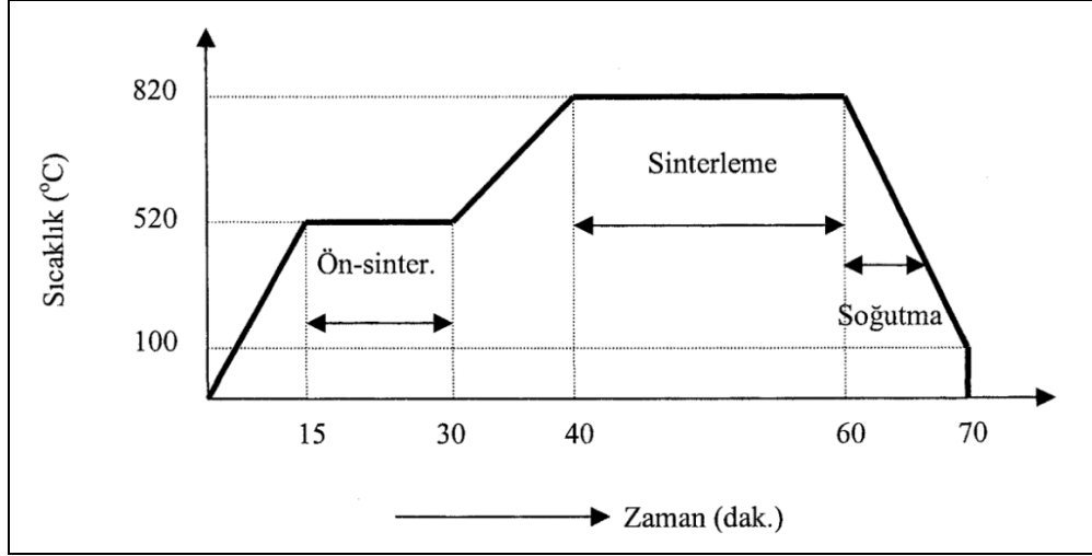
Şekil 4.9 Sinterleme işleminin aşamaları
