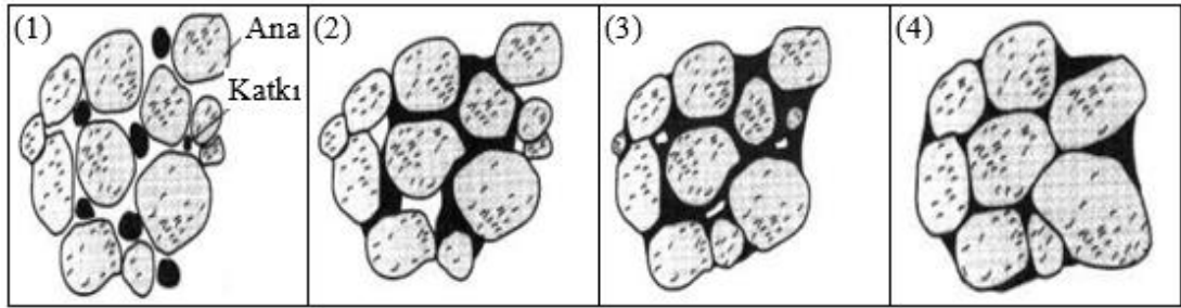
Şekil 4.14 İki toz karışımı kullanarak sıvı faz sinterlemesinin aşamaları
