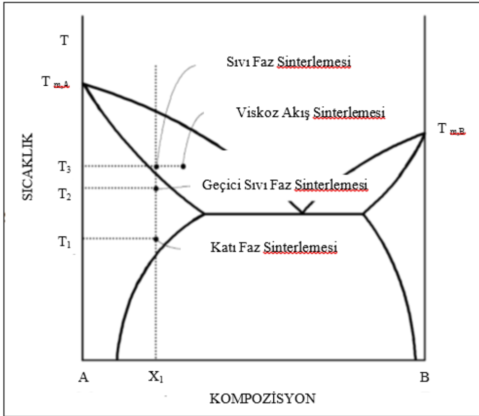
Şekil 4.13 Sinterleme faz diyagramı (Suk-Joong vd., 2005)
