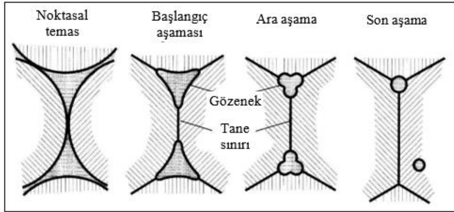
Şekil 4.12 Sinterleme esnasında gözenek yapısının değişiminin şematik resim
