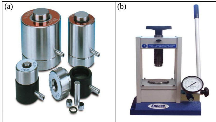
Şekil 5.1 a) kalıp b) Specac GS15011 marka pelet cihazı
