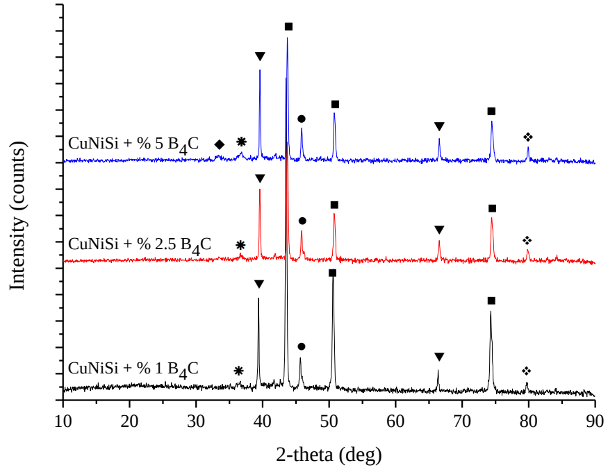
Şekil 6.12 Farklı oranlarda B 4 C takviyeli üretilen CuNiSi kompozit numunelerinin XRD grafikleri
