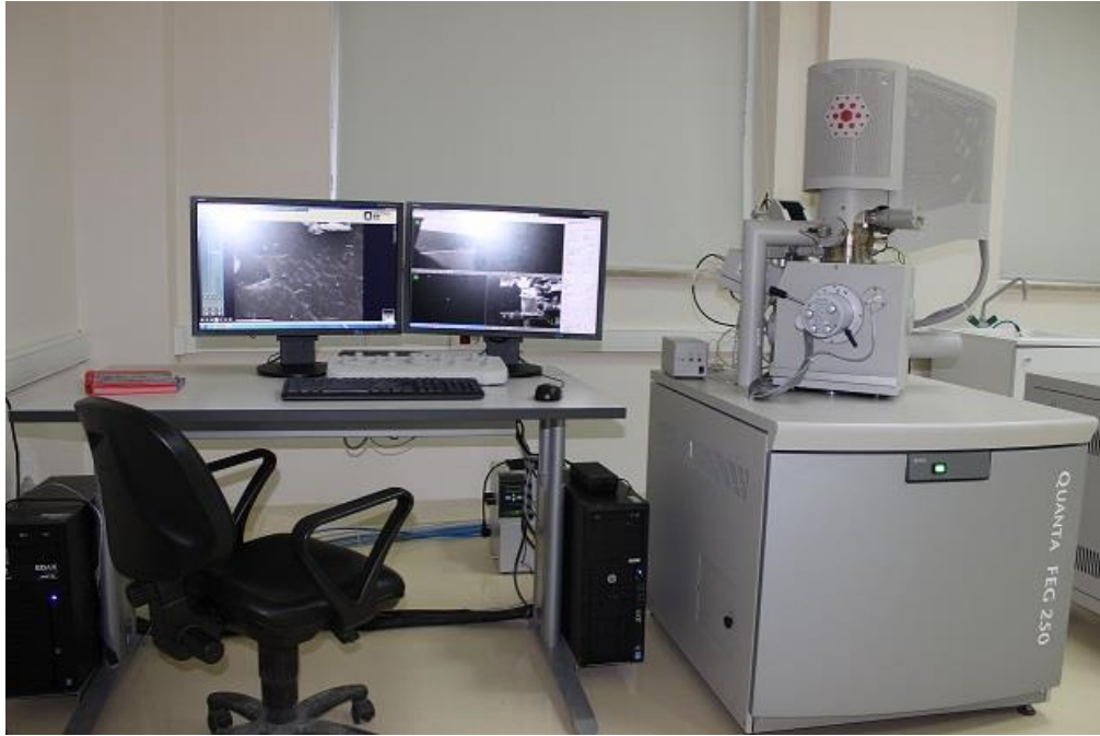
řekil 5.3 FEI QUANTA 250 FEG marka SEM analiz cihazı
