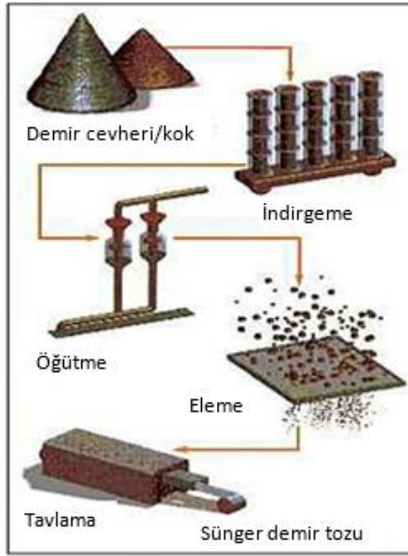
Şekil 3.4 Kimyasal yöntemle demir tozu imalatı
