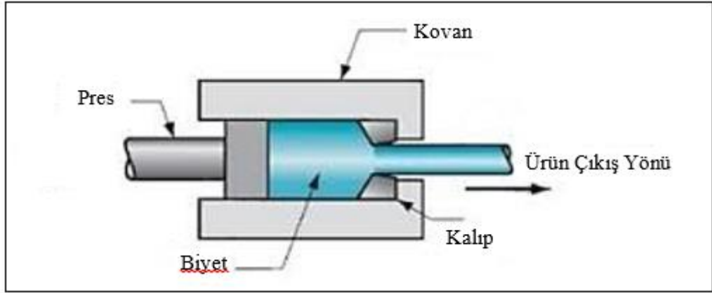
Şekil 4.3 Ekstrüzyon işleminin şematik gösterimi
