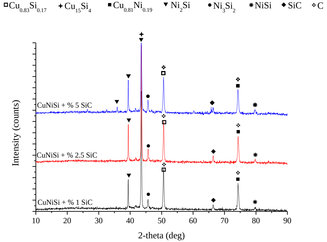
Şekil 6.13 Farklı oranlarda SiC takviyeli üretilen CuNiSi kompozit numunelerinin XRD grafikleri
