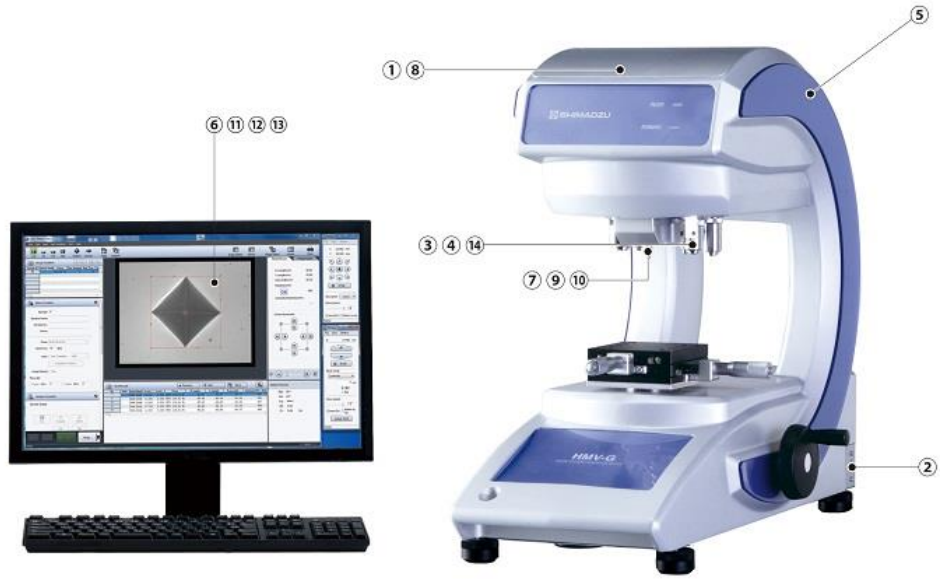
Şekil 5.5 SHIMADZU marka HMV-G21 model mikrosertlik ölçüm cihazı
