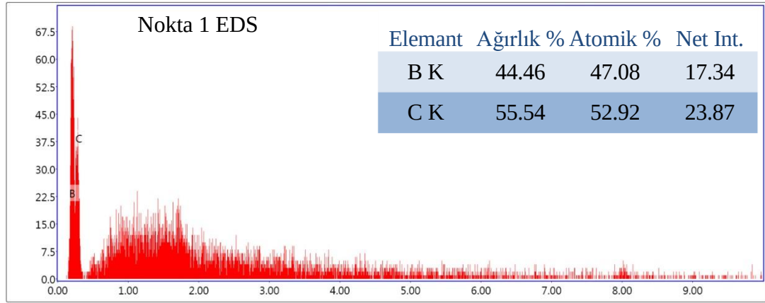
Şekil 6.7 Üretilen %5 B 4 C takviyeli CuNiSi kompozitinin SEM-EDS analiz sonucu
