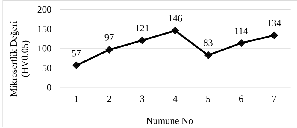
Şekil 6.14 Üretilen numunelerin mikrosertlik değerleri
