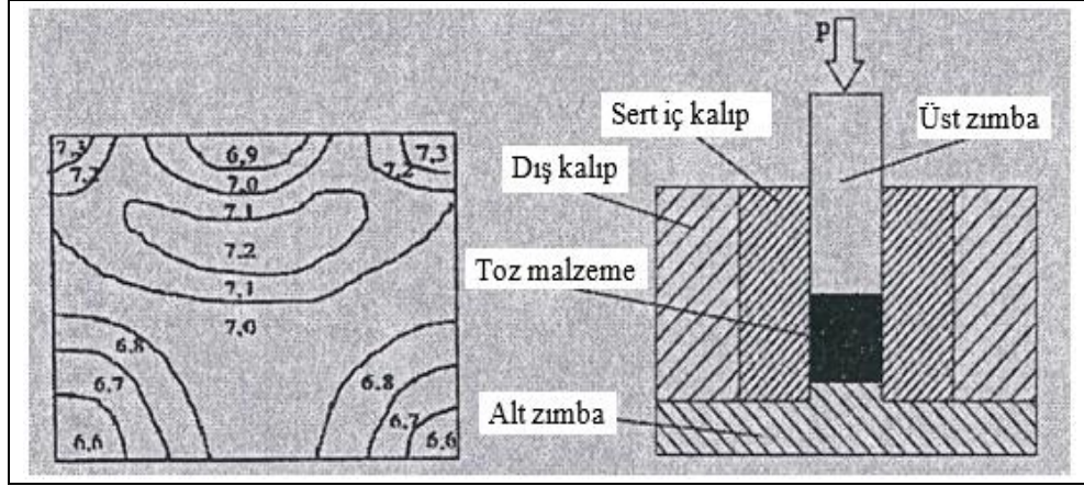
Şekil 4.5 Tek yönlü preslemede yoğunluk dağılımı ve tek yönlü kalıbın şematik gösterimi (Bahçeci, 2006; Matik, 2010)
