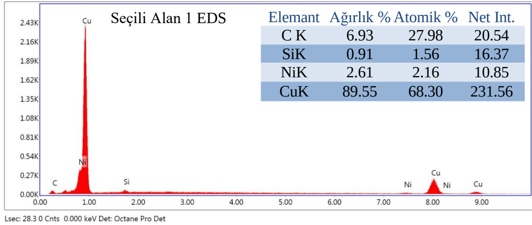
Şekil 6.9 Üretilen %2,5 SiC takviyeli CuNiSi kompozitinin SEM-EDS analiz sonucu
