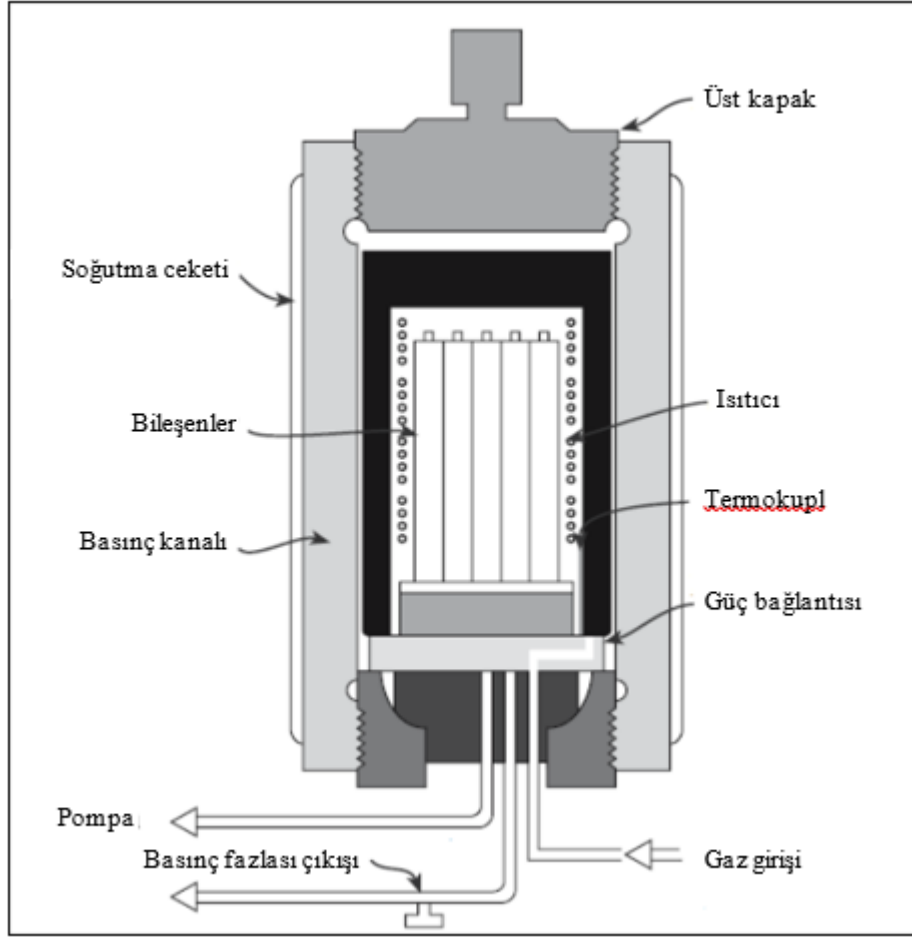
Şekil 4.8 Sıcak izostatik presleme şematik gösterimi (Matik, 2010)
