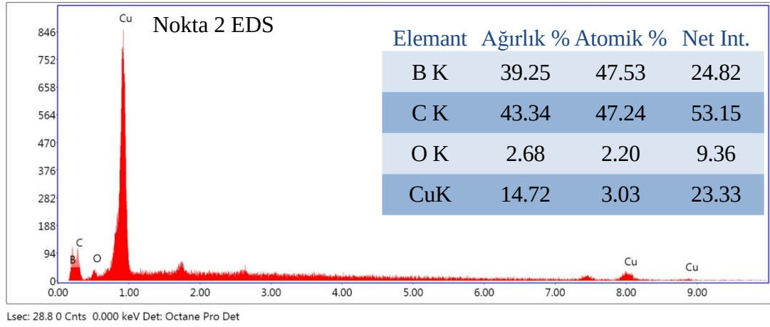
Şekil 6.5 Üretilen %1 B 4 C takviyeli CuNiSi kompozitinin SEM-EDS analiz sonucu
