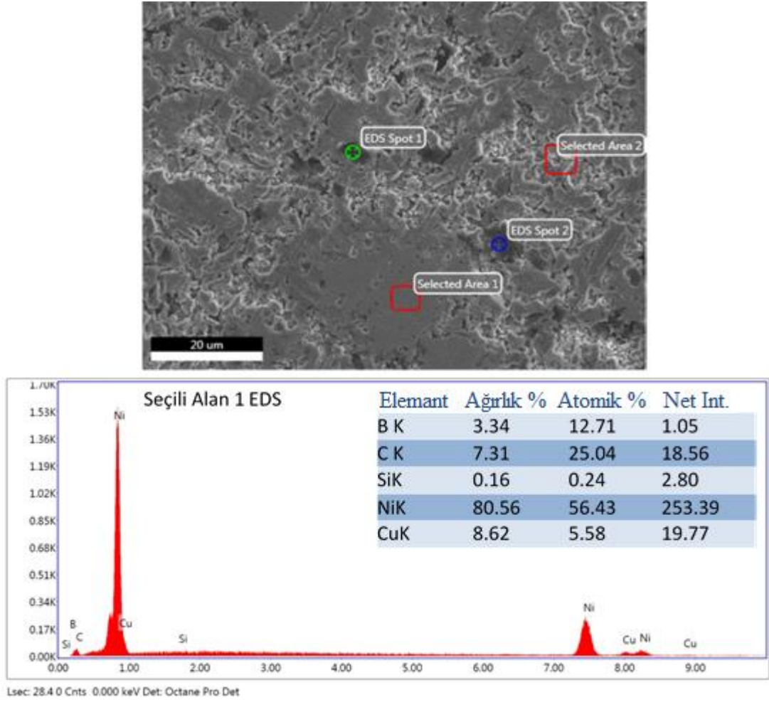
Şekil 6.6 Üretilen %2,5 B 4 C takviyeli CuNiSi kompozitinin SEM-EDS analiz sonucu
