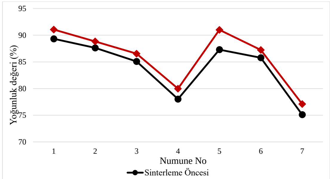
Şekil 6.15 Numunelerin yoğunluk değerleri
