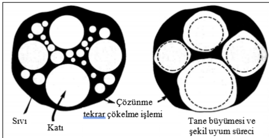
Şekil 4.15 Sıvı faz sinterleme işleminde çökeltme ve tane büyümesi
