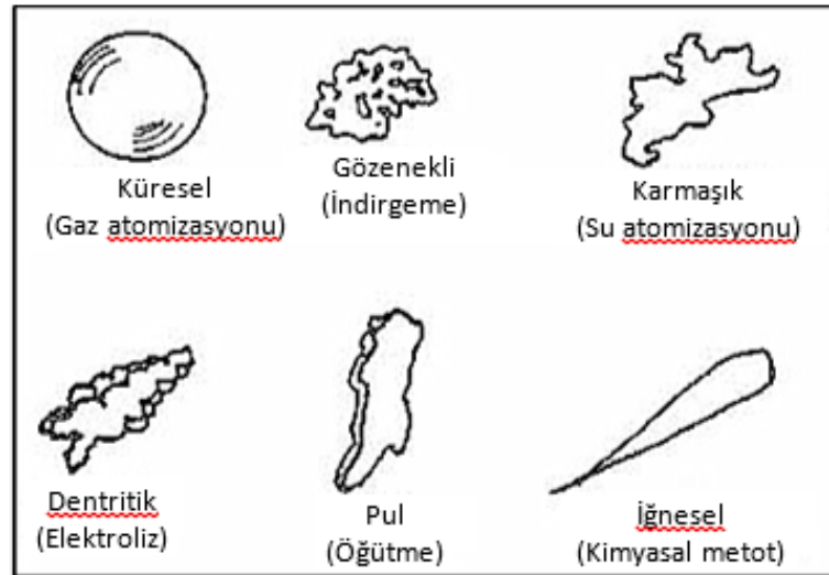
Şekil 3.3 Üretim metotlarına göre toz şekilleri (Yaşa, 2008)
