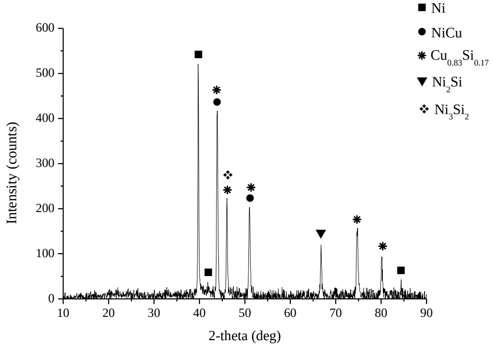
Şekil 6.11 Üretilen CuNiSi kompozit numunenin XRD grafiği
