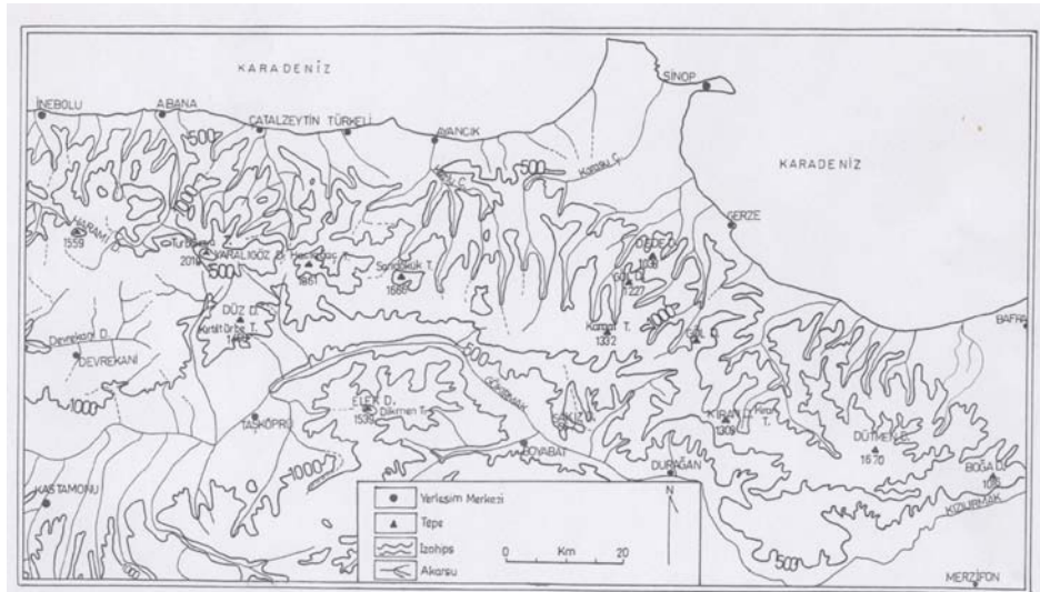
Şekil 2. İnceleme Sahasının Topografya Haritası. Figure 2. The Topografic Map of Research Area.
