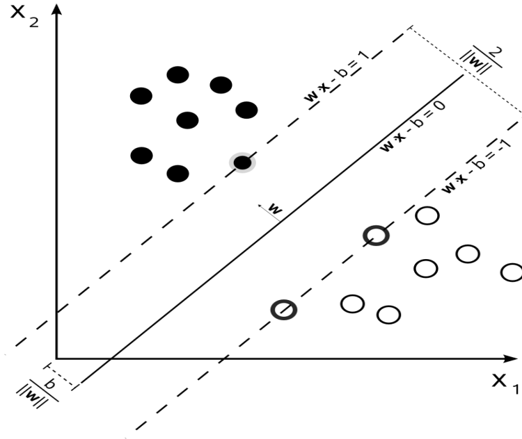
Şekil 4. 5. SVM Sınıflandırması
