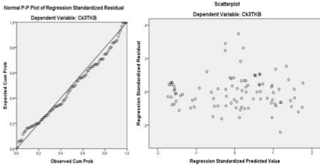
Şekil 4.7. Çk3KBT için dağılım grafikleri
