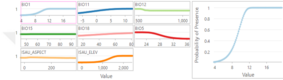
Şekil 4.137 İsaurica potansiyel alanlarında iklimsel değişkenlere ait grafikler
