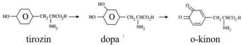
Şekil 1.2. Tirozinin kinona dönüştürülmesi.
