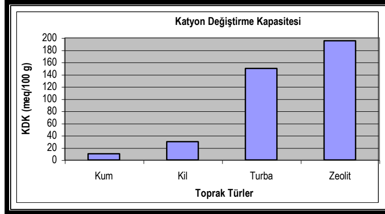
Şekil: 2 - Bazı Toprak Türleri ve Zeolitlerin Katyon Değişirme Kapasiteleri (Anonim, 2001c)
