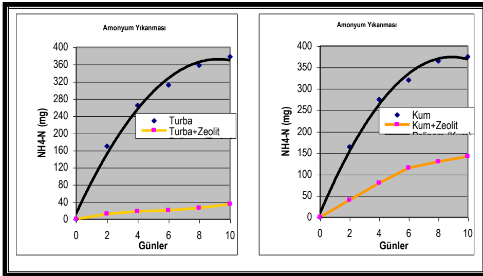
Şekil: 3 - NH 4 + İyonlarının Yağmur ve Sulama Suları ile Yıkanması (Anonim, 2001c)
