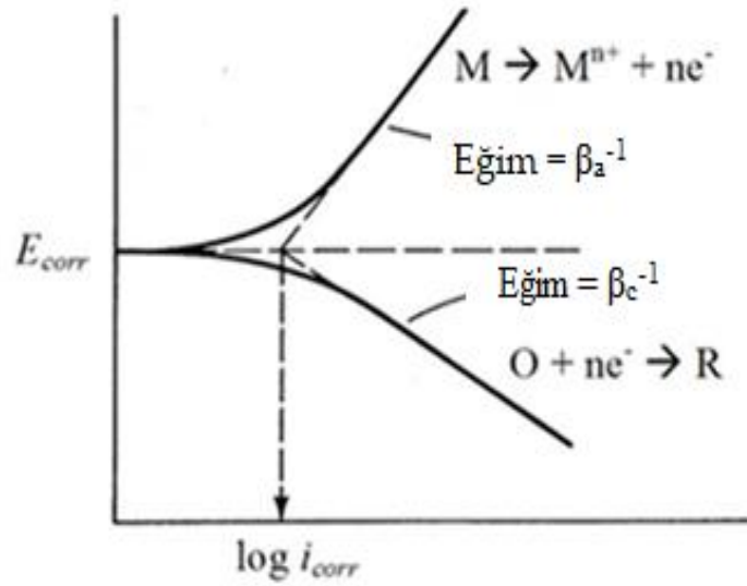
Şekil 1.10. Tafel bölgelerinin ekstrapolasyonunu gösteren toplam akıma karşı potansiyel eğrisi
