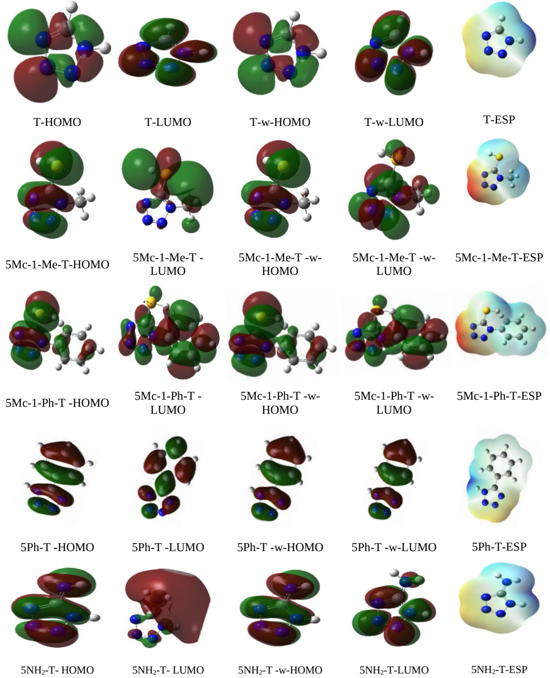
Şekil 4.25. Tetrazol türevlerinin nötr ve su fazındaki HOMO, LUMO ve toplam yük yoğunluğu
