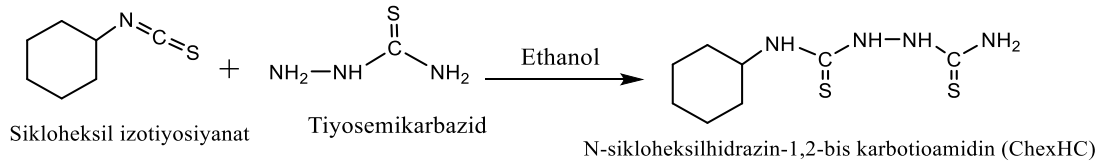
Şekil 3.3. ChexHC'nin sentez reaksiyonu
