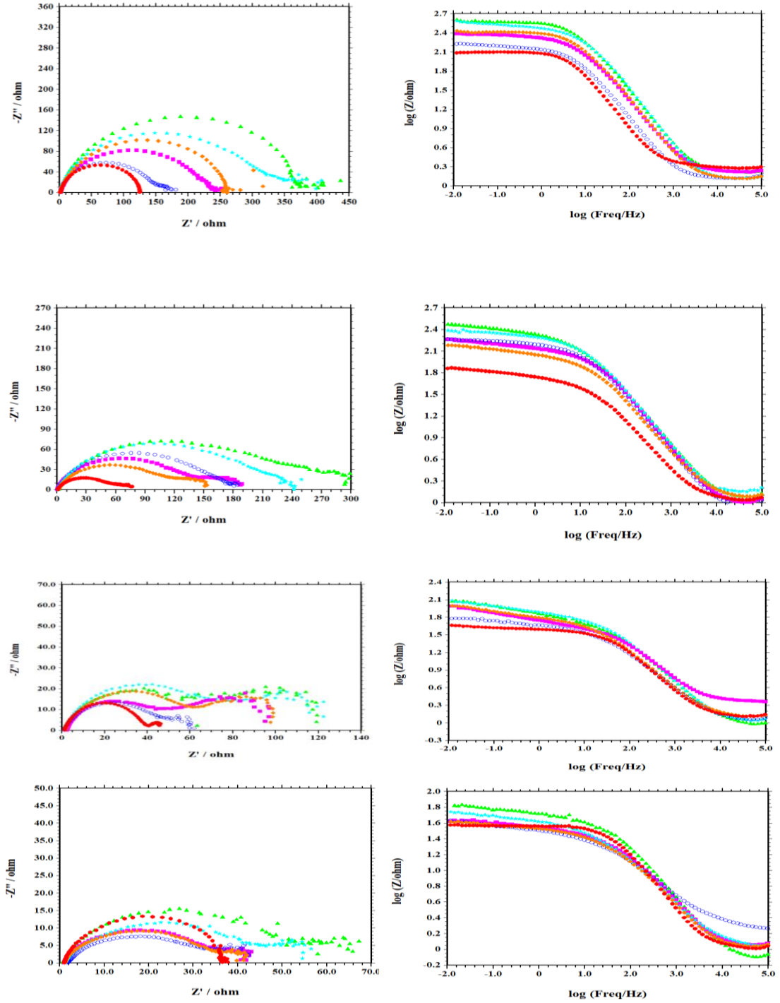
Şekil 4.6. 1,0 M HCl (●), 1,0x10 -5 M (○), 5,0x10 -5 M (■), 1,0x10 -4 M (■), 5,0x10 -4 M (★) ve 1,0x10 -3 M (▲) 2F-PhenHC çözeltilerinde 298, 308, 318 ve 328 K’de yumuşak çeliğin Nyquist ve Bode eğrileri
