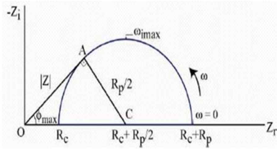
Şekil 1.8. Devrenin Empedans Nyquist grafiği
