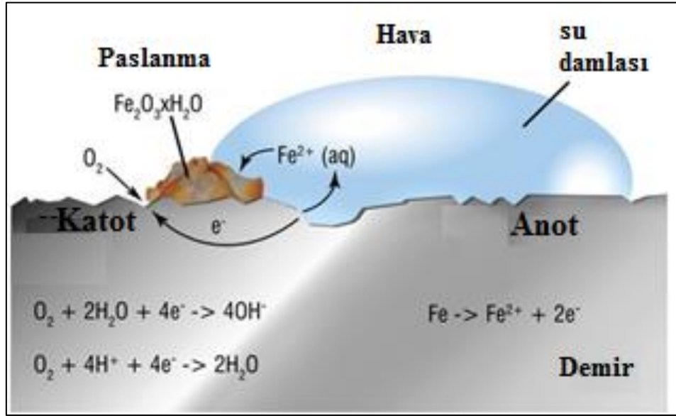
Şekil 1.1. Demirin oksidasyon reaksiyonu (McCafferty, vd., 2010)
