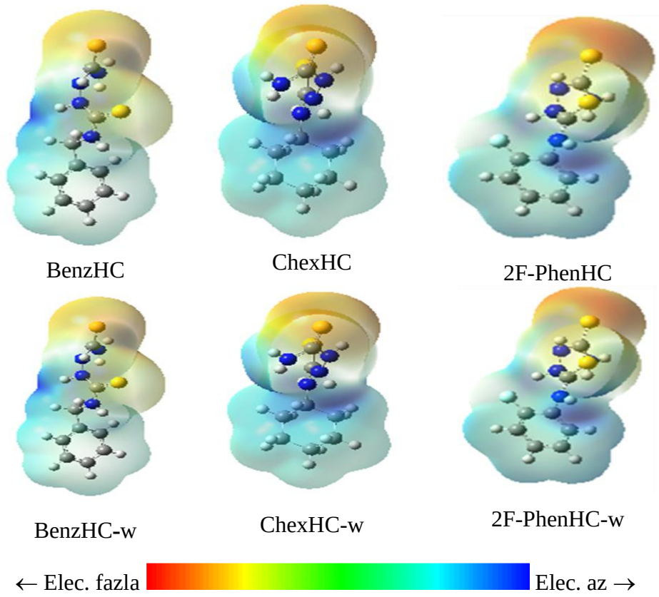
Şekil 4.22. Gaz ve su fazı için BenzHC, ChexHC ve 2F-PhenHC'nin elektron yoğunlukları
