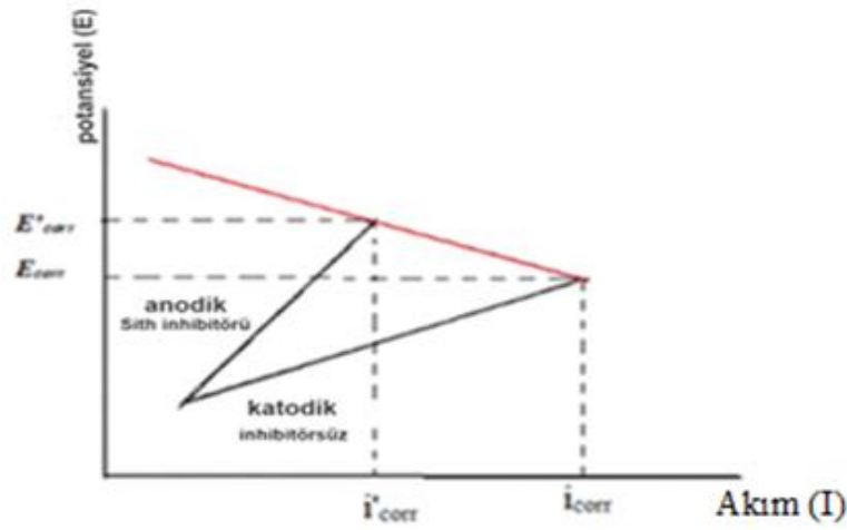
Şekil 1.4. Anodik inhibitörün Tafel eğimine etkisi
