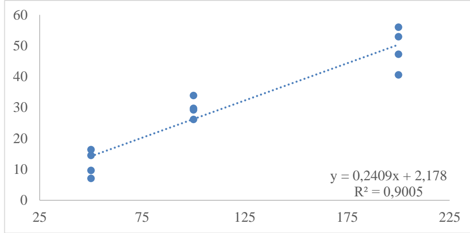
Şekil 4.3 Vitamin C % serbest radikal süpürme etkisi
