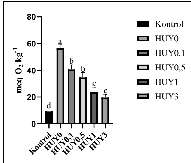
Şekil 4.4 Deney gruplarının termal oksidasyon uygulanmış balık yağı üzerindeki koruyucu etkisi
