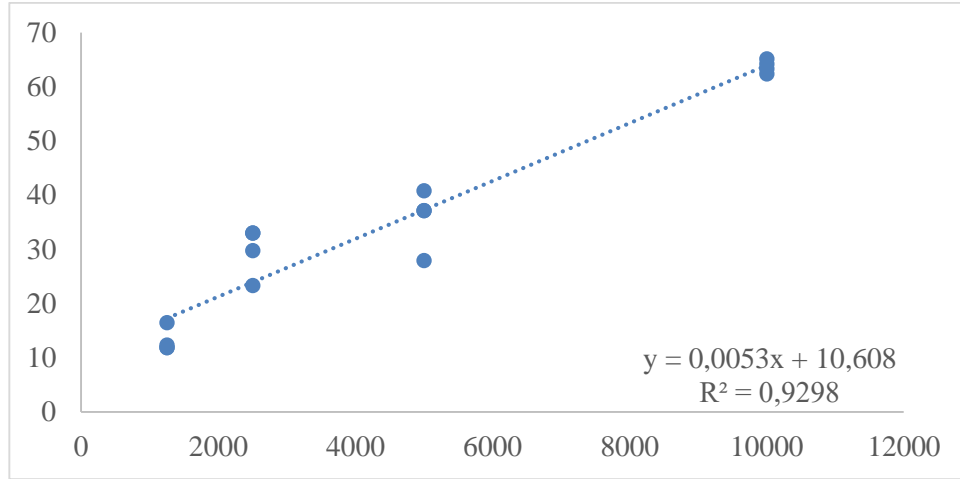
Şekil 4.1 HUY % serbest radikal süpürme etkisi
