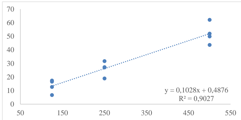
Şekil 4.2 BHT % serbest radikal süpürme etkisi
