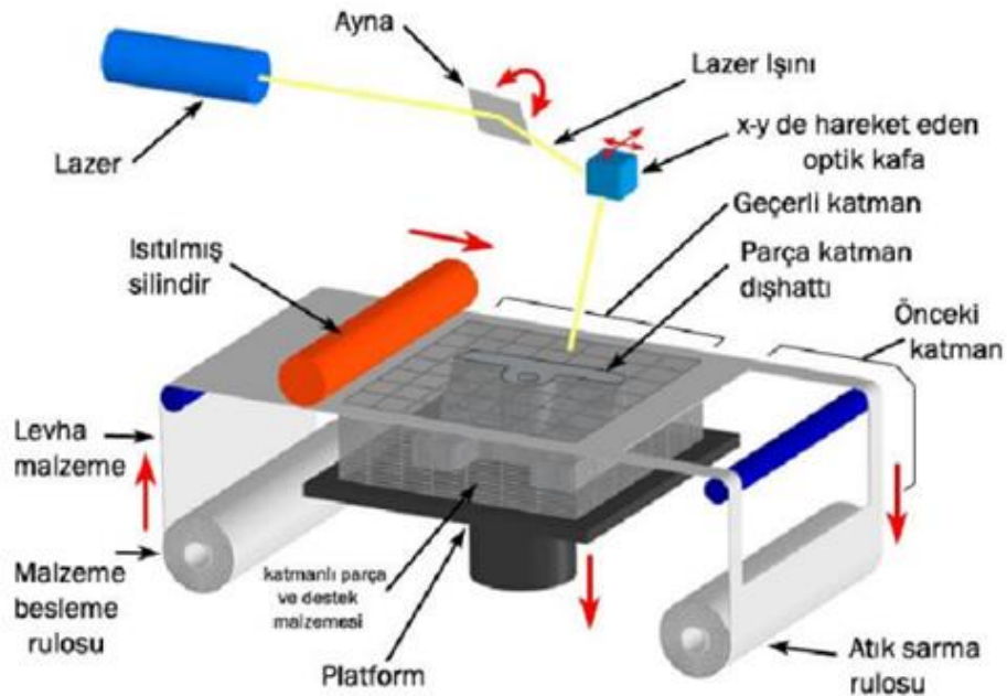
Şekil 2.25 LOM çalışma düzeneği
