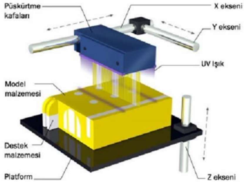
Şekil 2.24 Polijet çalışma düzeneği
