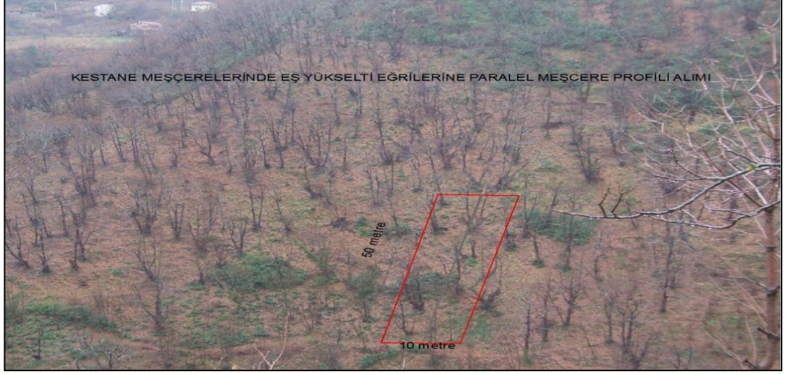
Şekil 3.9. Eş yükselti eğrilerine paralel alınan meşcere profilleri
