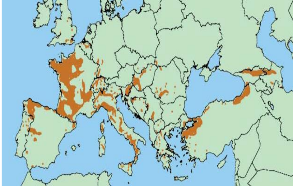
Şekil 3. 1. Anadolu keşanesi ( Castanea sativa Mill.) nin Dünyadaki doğal yayılış alanları
