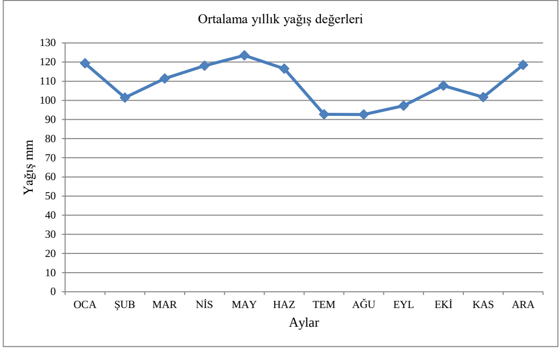
Grafik 3.2. Keltepe mevki enterpole edilmiş ortalama yıllık yağış değerleri
