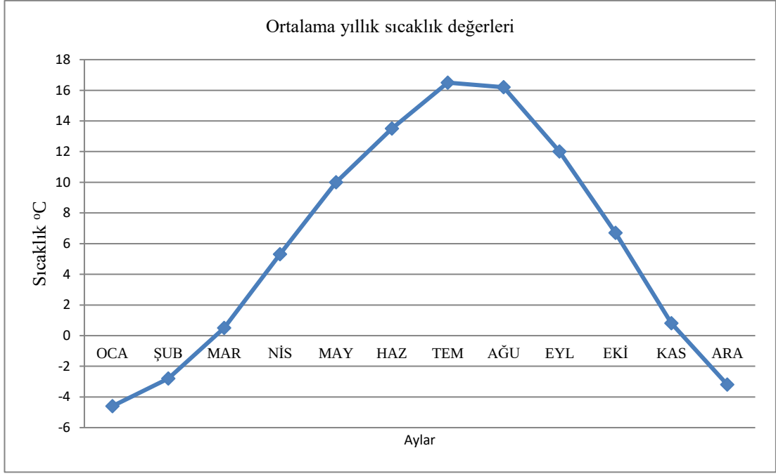
Grafik 3.1. Keltepe mevki enterpole edilmiş ortalama yıllık sıcaklık değerleri
