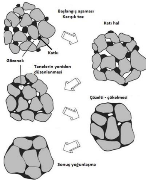
Şekil 4.4. Sıvı faz sinterleme mekanizmasının aşamaları (Cengiz, 2016)
