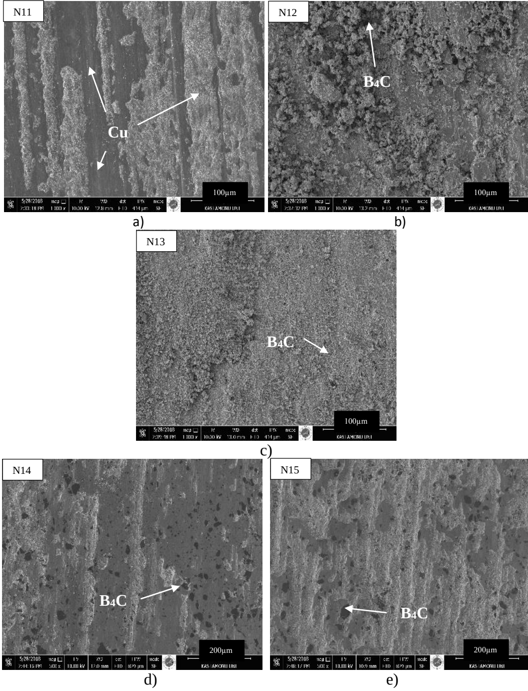
Şekil 8.26. 850 0 C’de sinterlenen farklı takviye oranlarına sahip kompozitlerin aşınma görüntüleri a) Saf bakır b) %2,5 B 4 C c) %5 B 4 C d) %7,5 B 4 C e) %10 B 4 C
