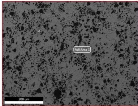
N08 (%95,0 Cu - %5,0 B 4 C) numunesine ait mikroyapı görüntüsü ve EDS analizi
