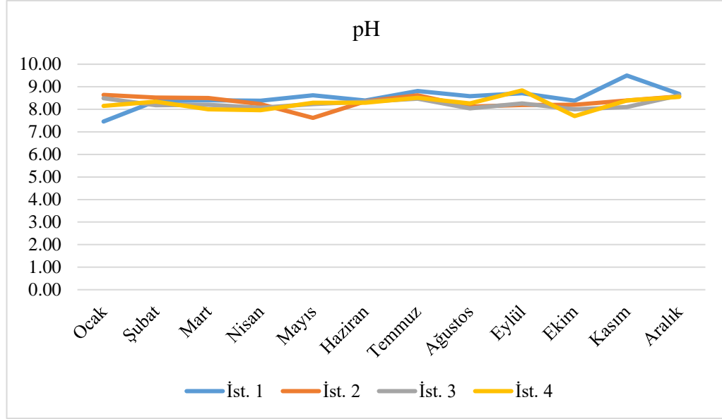
Grafik 4.2. İstasyonlara göre pH'nin aylık değişimi
