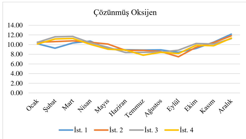
Grafik 4.4. İstasyonlara göre çözünmüş oksijen düzeyinin ( \text{mg l}^{-1} ) aylık değişimi
